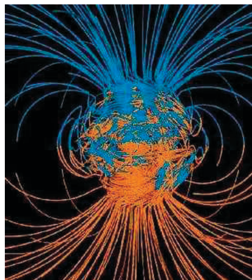
科學家們證實地球的兩極有時會出現大幅度的轉變。圖為計算機模擬演示的地球的磁場。
