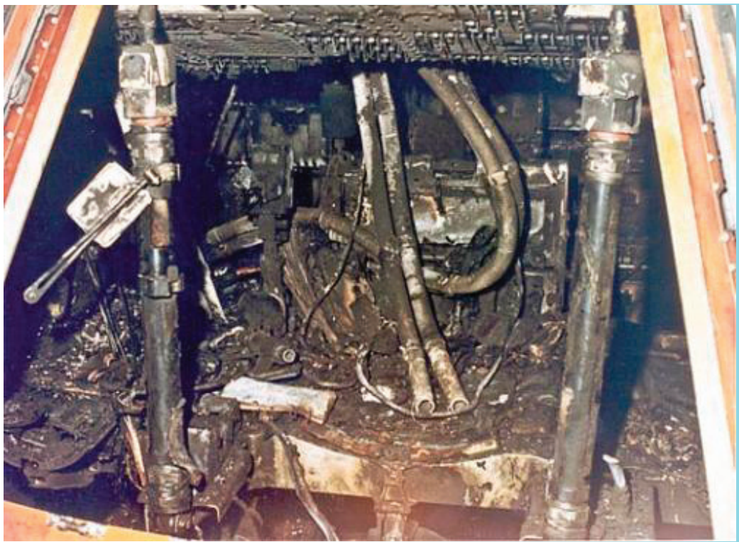
密封指令艙因意外事故發生火災的「阿波羅一號」殘骸
